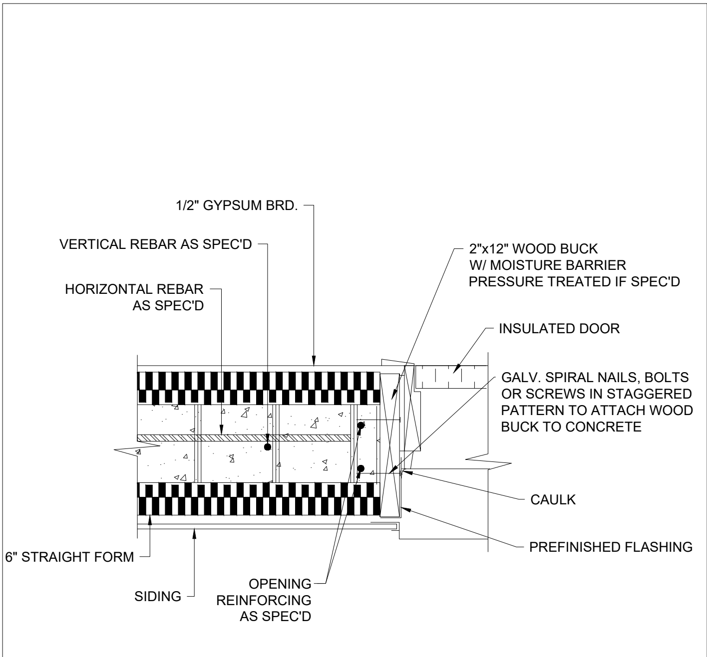
1 DOOR JAMB DETAIL 6 INCH
